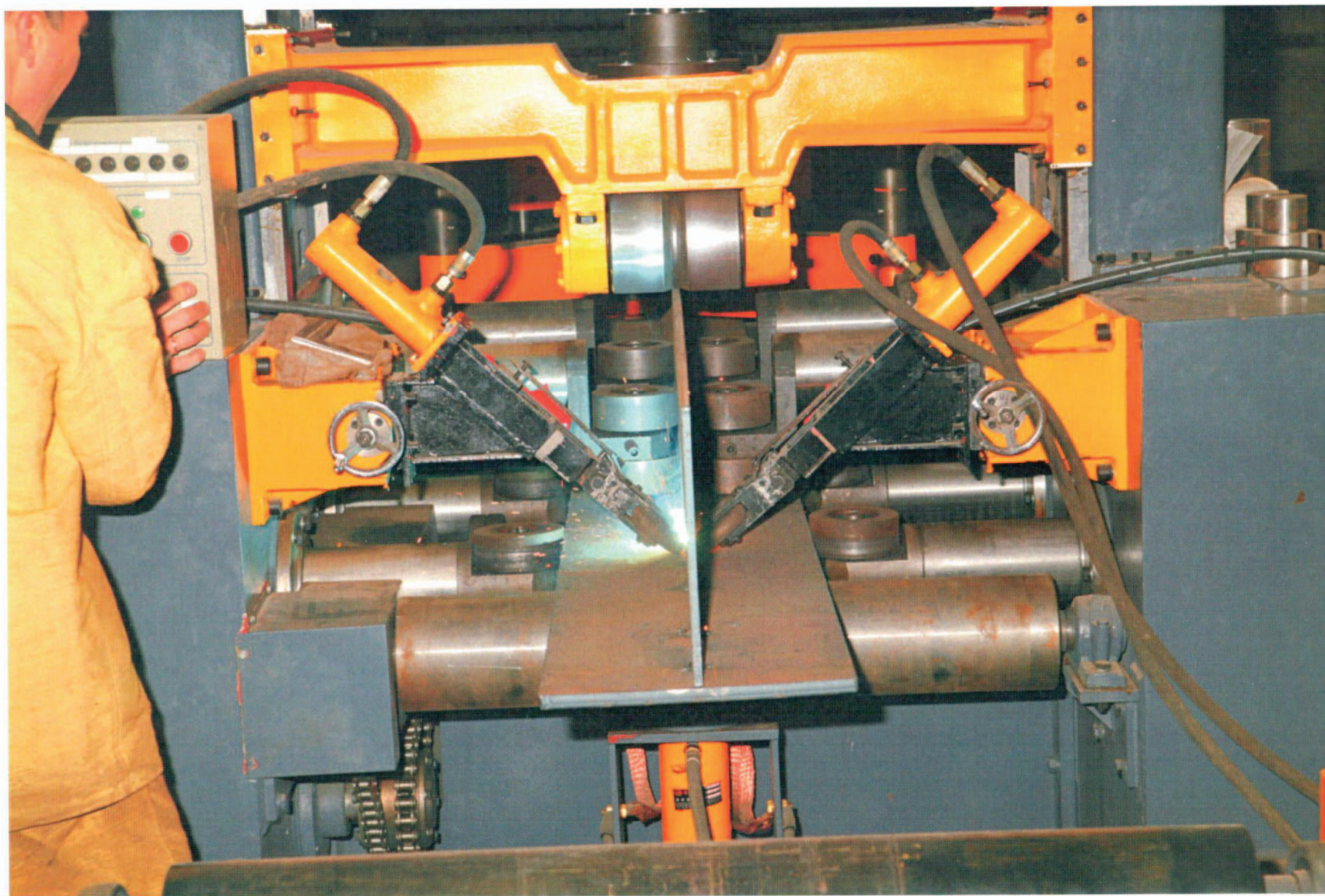
Стан сборки двутавровой балки
