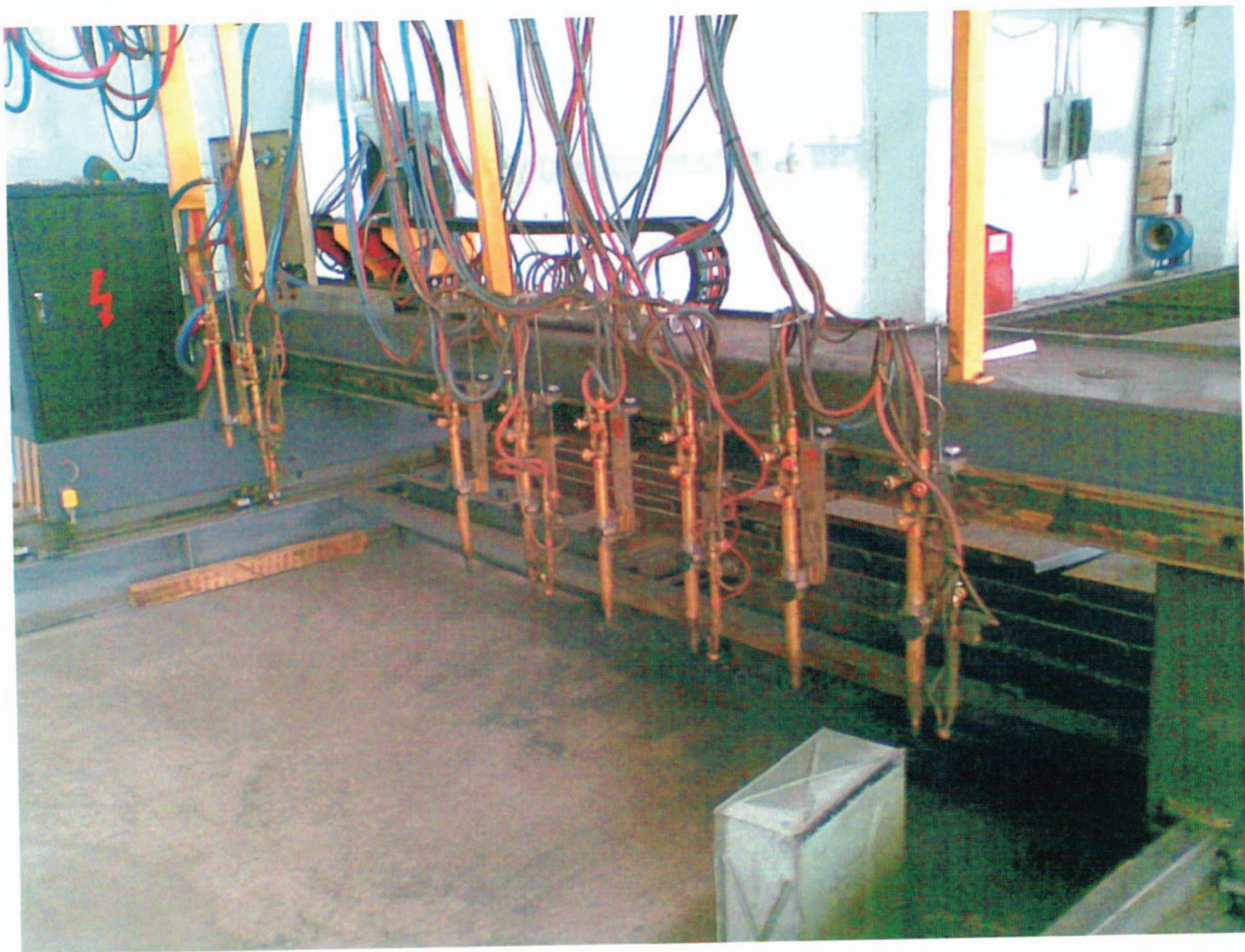
Машина термического раскроя листового проката OSG Machinery Co. с восемью резаками
