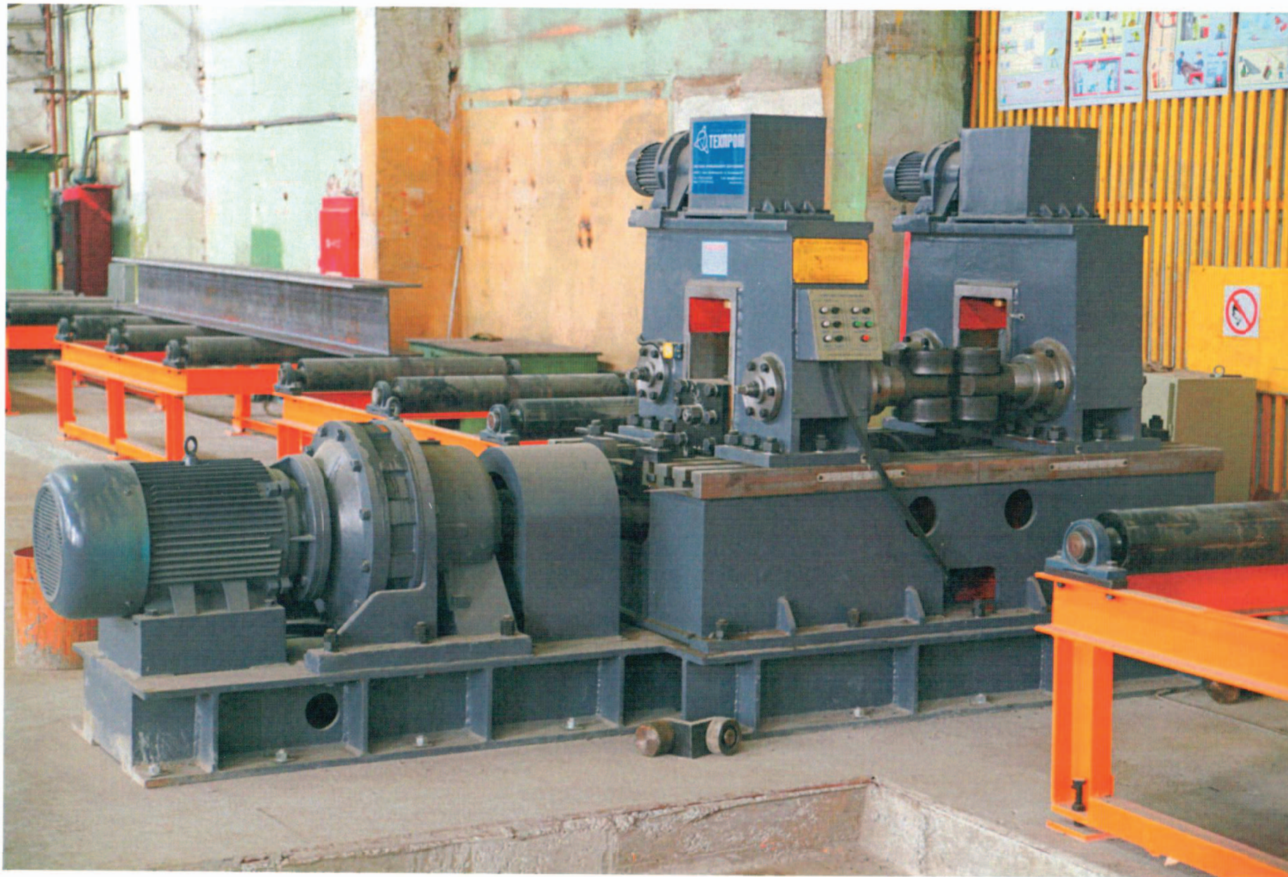
Стан правки грибовидности полков двутавровой балки
