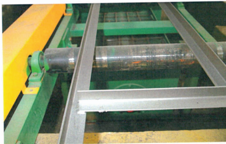
Конструкции после дробеметной очистки (класс очистки Sa-3)
